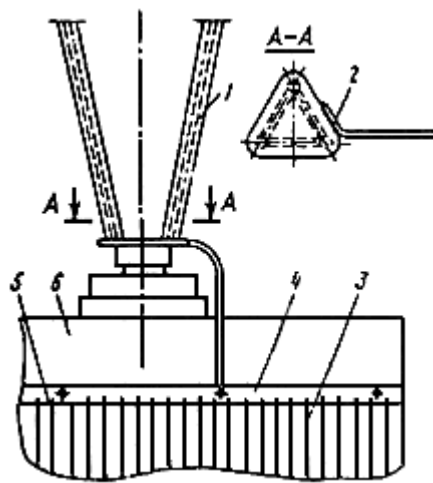
Рис.4. Молниезащита мачты, неизолированной в основании
