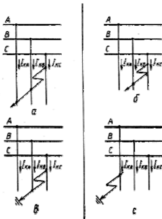
а - трехфазное КЗ - K^{(3)} ; б - двухфазное КЗ - K^{(2)} ; в - двухфазное КЗ на землю - K^{(2,1)} ; c - однофазное КЗ на землю - K^{(1)}
