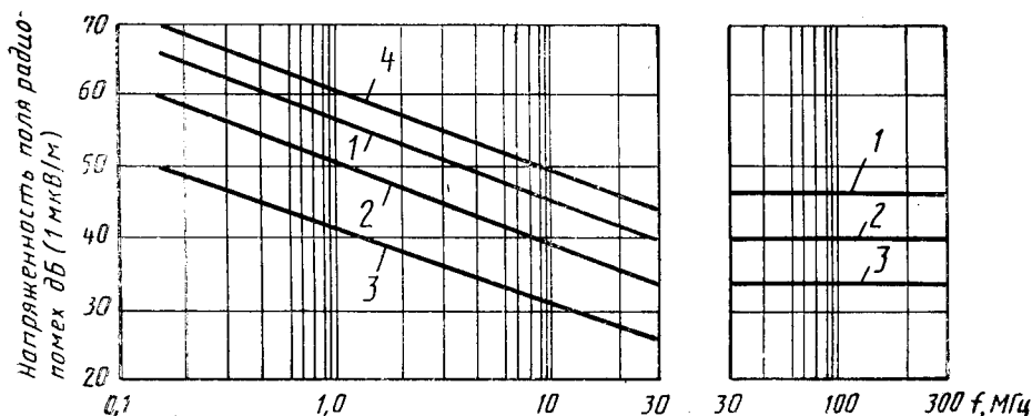
Нормы напряженности поля радиопомех
