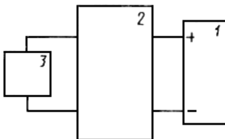
1 - испытуемое изделие; 2 - имитатор помех; 3 - блок питания
