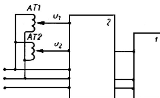
1 - испытуемое изделие; 2 - имитатор помех; AT1 , AT2 - автотрансформаторы
