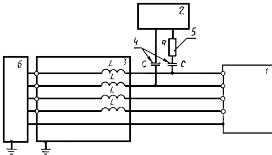
1 - испытуемое изделие; 2 - генератор; 3 - разделительное устройство; L = 1,5 мГн; 4 - конденсаторы связи, C = 0,5 мкФ (2 шт.); 5 - сопротивление связи, R = 40 Ом; 6 - внешнее устройство
