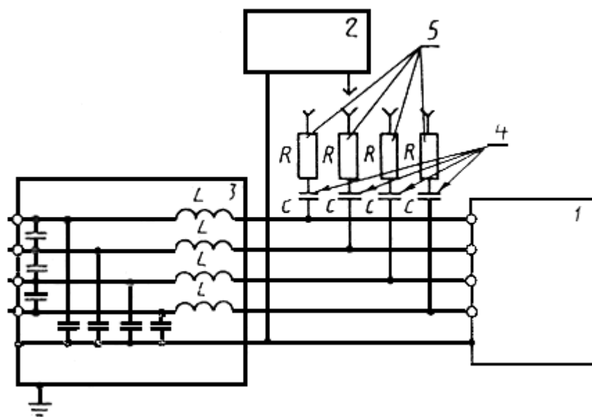
1 - испытуемое изделие; 2 - генератор; 3 - разделительное устройство; 4 - конденсатор связи, C = 9 мкФ (4 шт.); 5 - сопротивление связи, R = 10 Ом (4 шт.)
