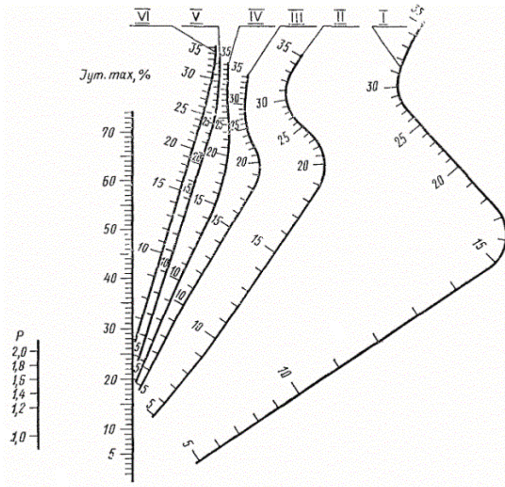
I, II, III, IV, V, VI - кривые номограммы с расстояниями между тяговыми подстанциями: I-при n от 0 до 2; II-при n от 3 до 7; III-при n от 8 до 12; IV - при n от 13 до 17; V - при n от 18 до 23; VI - при n более 23.
