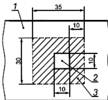
Рисунок И.2. - Схема проведения надреза для сдвига образца покрытия
