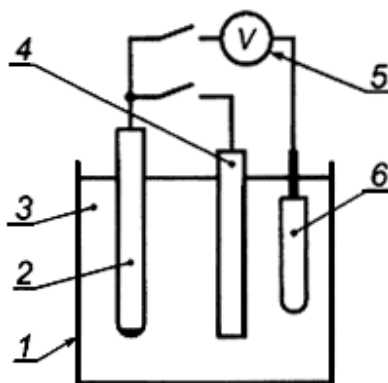
Рисунок Л.1 - Схема проведения испытания с применением магниевого анода
