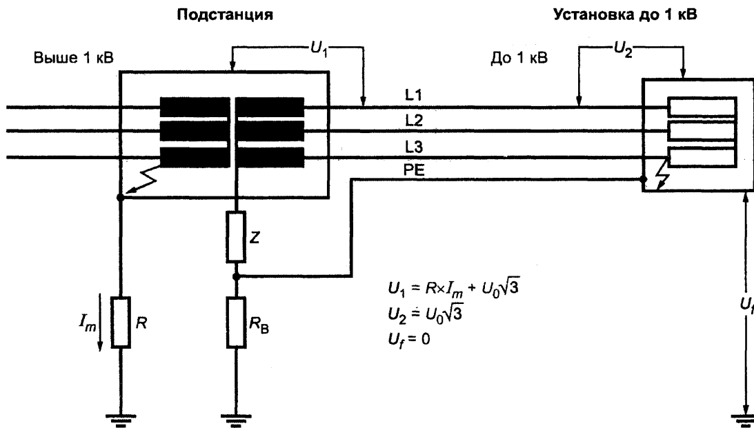
2) Первое замыкание в установке до 1 кВ
