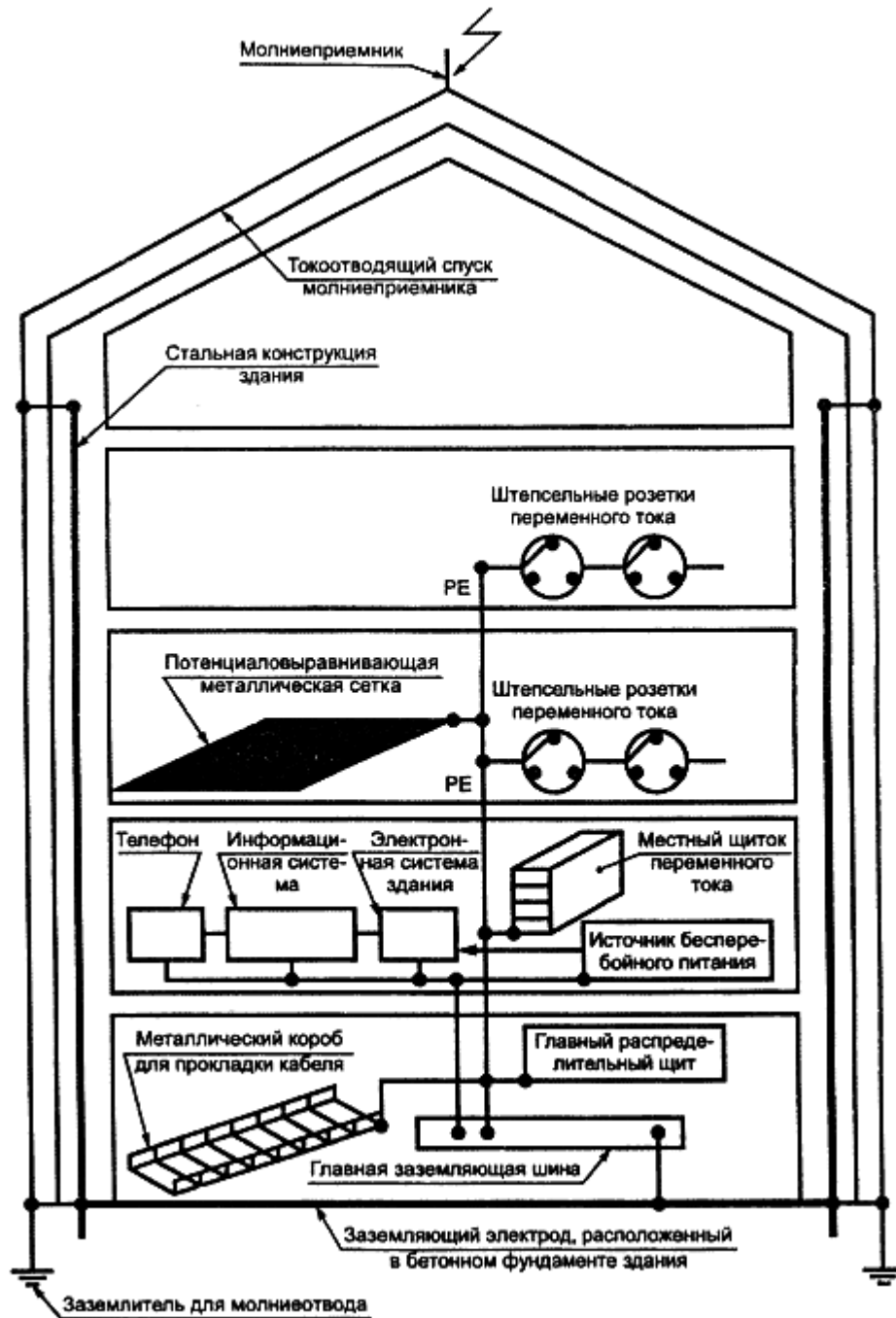
Рисунок 5 - Общий вид системы заземления здания в соответствии
