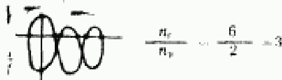
Рисунок 4 — Определение кратности частот по фигурам Лиссажу
