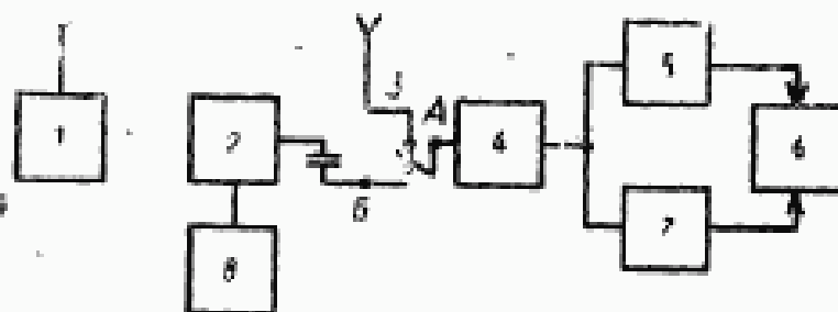
1 — проверяемый радиопередатчик; 2 — синтезатор частоты; 3 — переключатель; 4 — радиоприемник; 5 и 7 — полосовые фильтры, настроенные на первую и вторую гармоники основной частоты речевого спектра; 6 — осциллограф; 8 — электронно-счетный частотомер.
