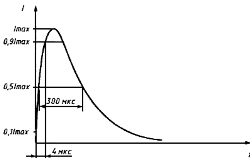
Рисунок 4 - Форма испытательного импульса при коротком замыкании ИГ
