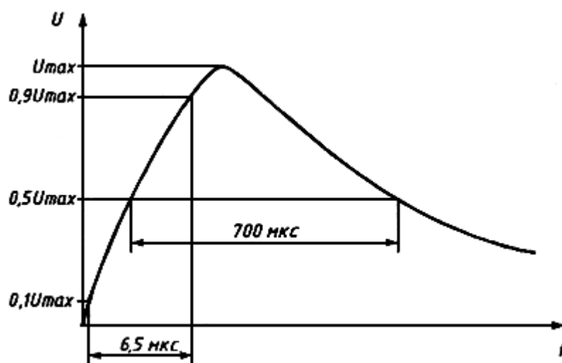
Рисунок 3 - Форма испытательного импульса при холостом ходе ИГ
