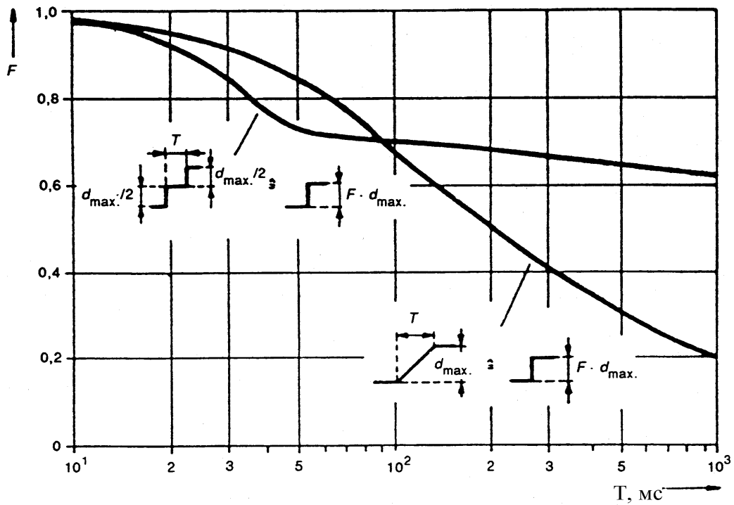
Рисунок 5 – Коэффициент приведения для двухступенчатых и линейно изменяющихся характеристик относительного изменения напряжения 14
