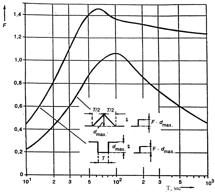
Рисунок 6 – Коэффициент приведения для прямоугольных и треугольных
