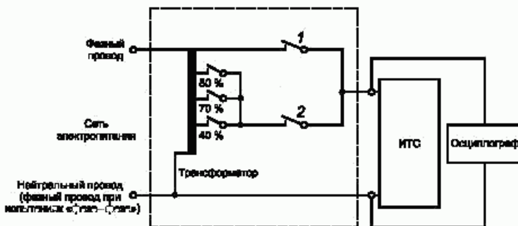
а) Схема испытаний с использованием трансформатора с отводами и переключателей
