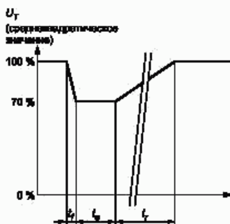
Рисунок 3 — Изменение напряжения
