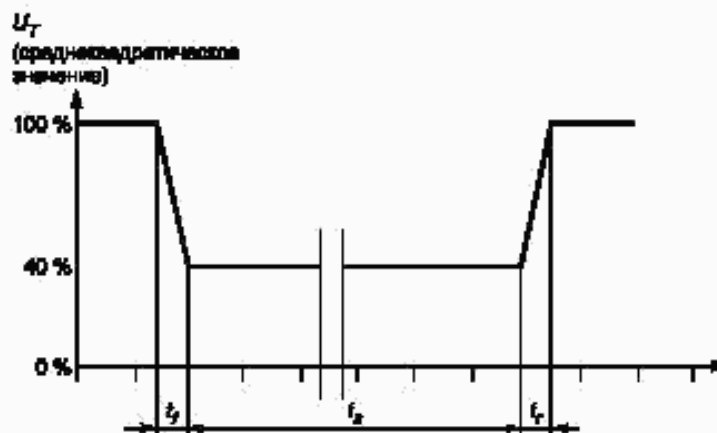
t_r — время нарастания напряжения; t_s — время понижения напряжения; t_f — время выдержки на пониженном напряжении
