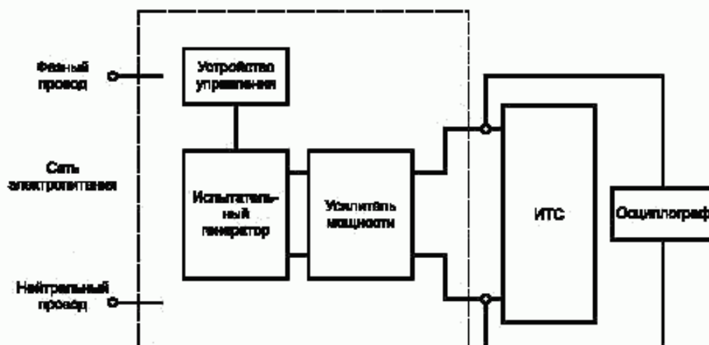
б) Схема испытаний с использованием усилителя мощности
