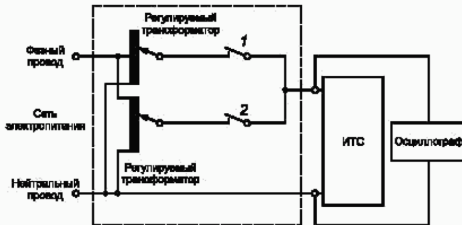
1, 2 — попеременно коммутируемые переключатели
