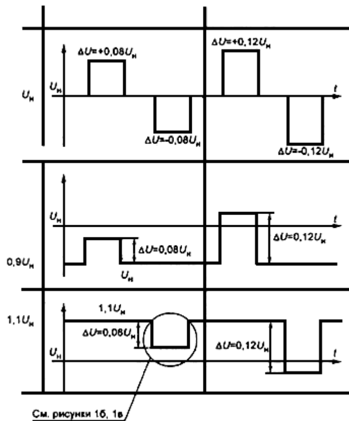
Рисунок 1а - Диаграмма колебаний напряжения
