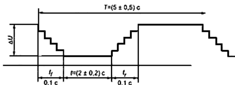
Рисунок 1б - Определение времени спада t_f и времени возрастания t_r при формировании ступенчатых изменений напряжения
