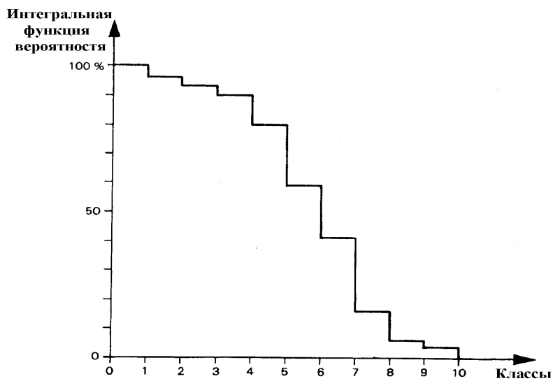
Рисунок 2б – Интегральная функция вероятности наличия сигнала а классах 1 - 10
