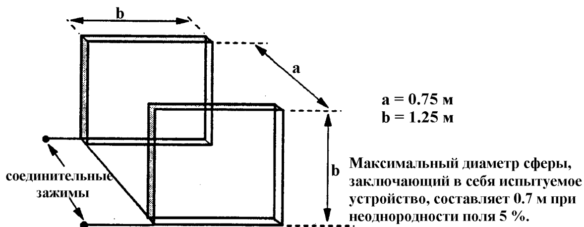
Рисунок А.1 – Конструкция катушки Гельмгольца для однородных полей
