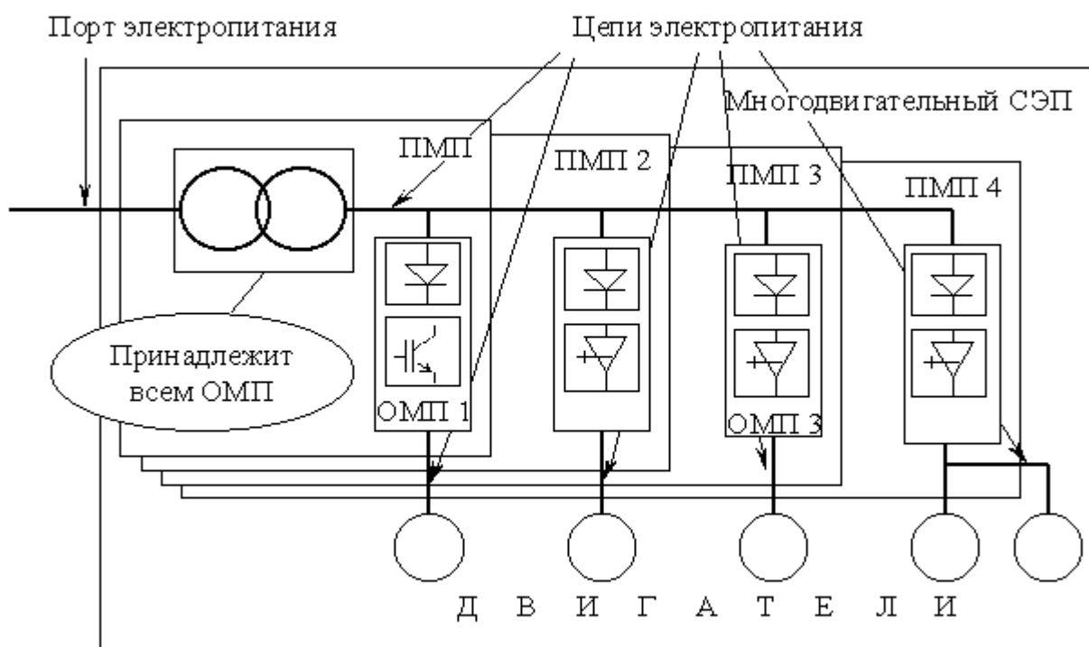
Рисунок 4 – Цепи электропитания СЭП с общим входным трансформатором
