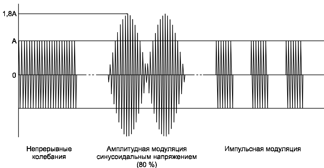
Рисунок 3 — Виды модуляции
