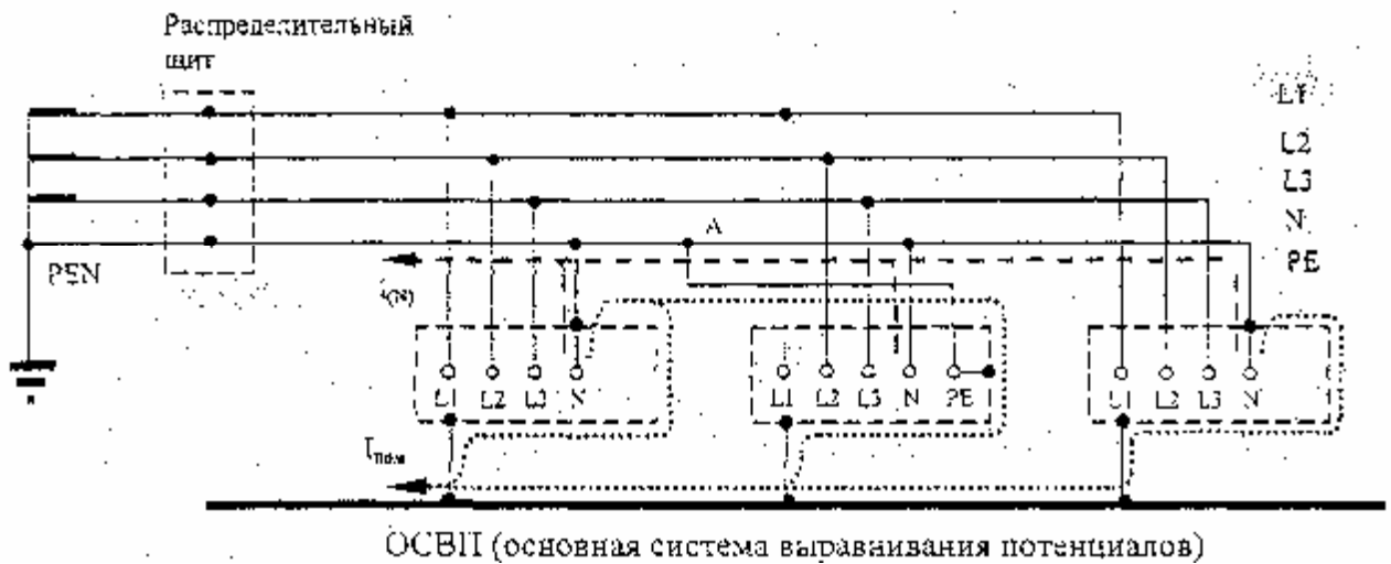
Рисунок Б.2 - Распределение токов проводников (N) при совмещении в одном фидере трехфазных четырехпроводной и пятипроводной систем проводников электропитающей сети переменного тока (за точкой, Д включается аппаратура с четырехпроводным и пятипроводным питанием)
