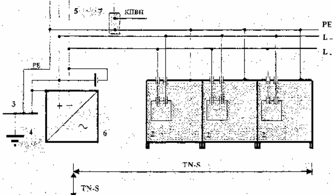
Рисунок 8 - Рекомендуемая схема заземления системы электропитания постоянным током аппаратуры ВОЛП в стоечном ряду для реконструируемых и действующих объектов
