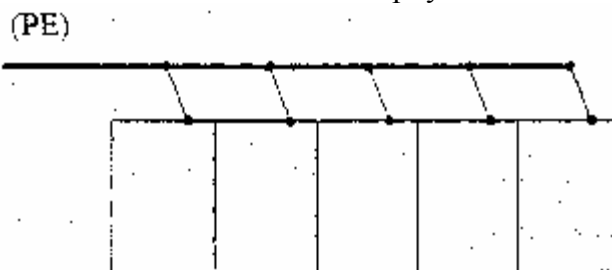
Рисунок 6 - Последовательно-параллельная схема заземления корпусов стоек аппаратуры ВОЛП
