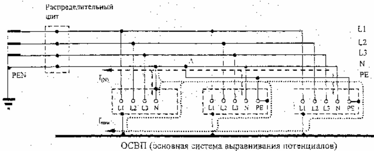
Рисунок 5.3 - Распределение токов проводников (N) и (PEN) при совмещении в одном фидере трехфазных четырехпроводной и пятипроводной систем проводников электропитающей сети переменного тока (за точкой А включается аппаратура только с пятипроводным питанием)
