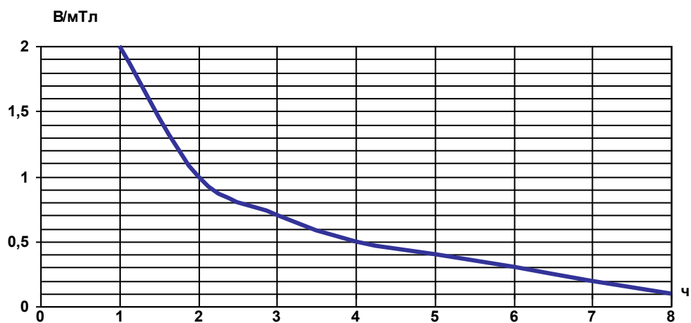
КРИВАЯ ИНТЕРПОЛЯЦИИ ПДУ МАГНИТНЫХ ПОЛЕЙ ЧАСТОТОЙ 50 Гц В ЗАВИСИМОСТИ ОТ ВРЕМЕНИ
