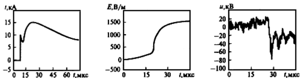
Рис.П.Е.2. Осциллограммы тока молнии, напряженности электрического поля молнии и напряжения наводки на воздушной линии
