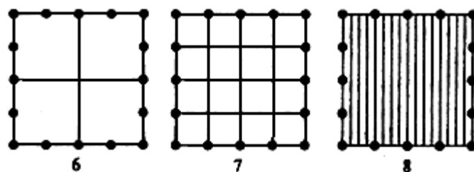
Рис.П.Е.1. Сложные заземлители
