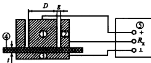
Рис.8. Схема измерений поверхностного и объемного сопротивления полимерного диэлектрика:
