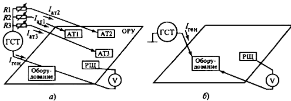
Рис.П.Д.1. Схема для имитации КЗ на высоковольтном оборудовании
