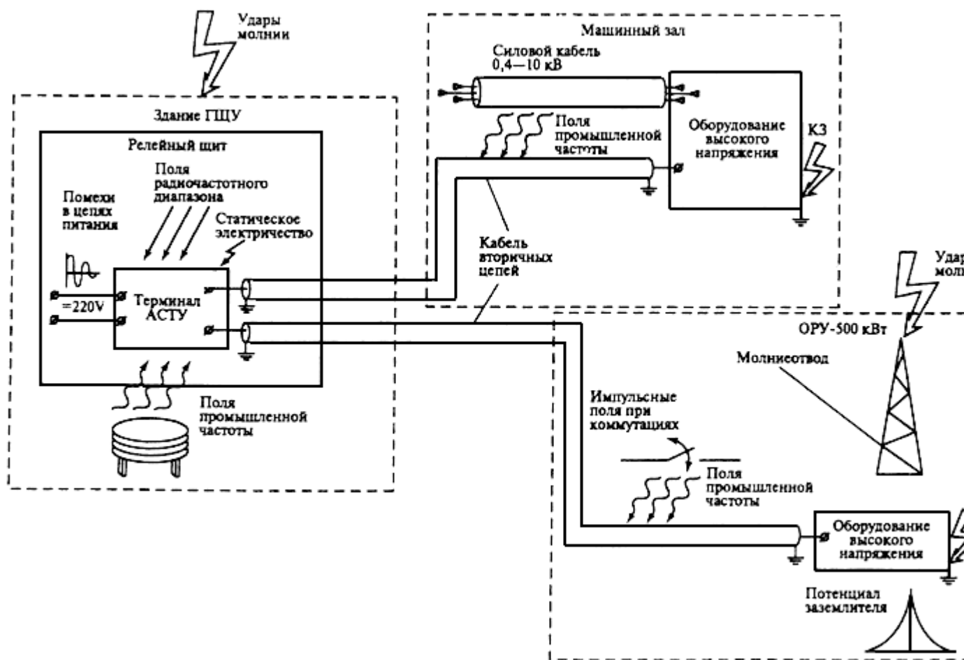
Рис.1. Источники электромагнитных помех:
