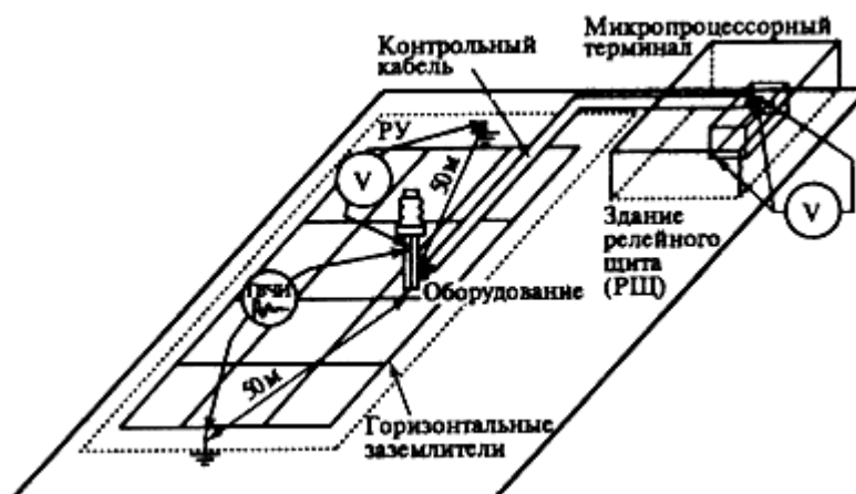
Рис.5. Схема эксперимента по определению импульсных помех при протекании высокочастотной составляющей тока КЗ
