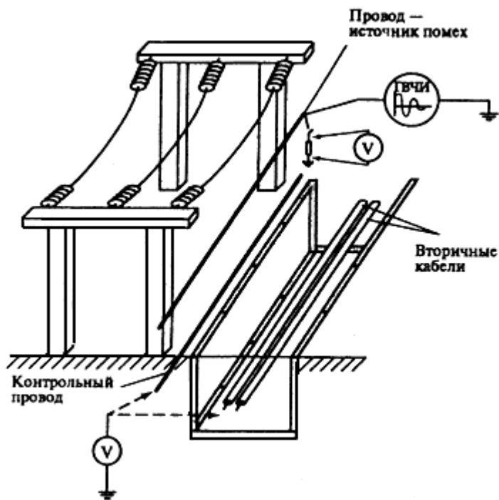
Рис.6. Схема имитации излучаемых помех
