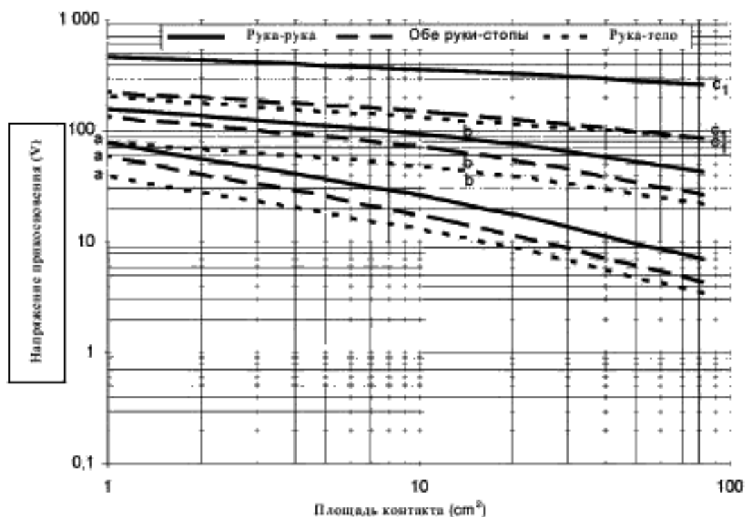
Рисунок 4 Минимум напряжения прикосновения при постоянном токе и сухих средах для тока вызывающего реакцию испуга(а), мышечную реакцию(б) и вентрикулярную фибрилляцию (с1)
