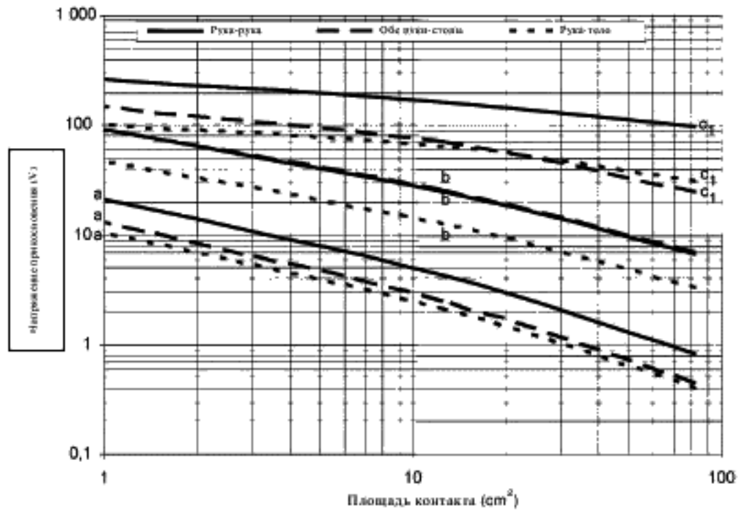
Рисунок 2 - Минимум напряжения прикосновения при переменном токе и влажных средах для тока вызывающего реакцию испуга (а), мускульную реакцию (b) и вентрикулярную фибрилляцию (c1)
