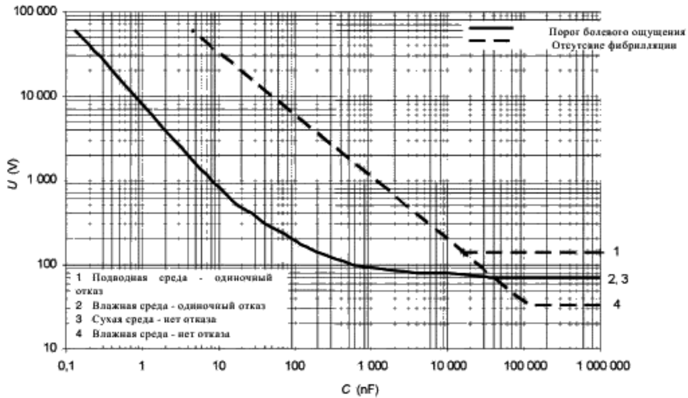
Рисунок А.1 - Параметры заряженных конденсаторов
