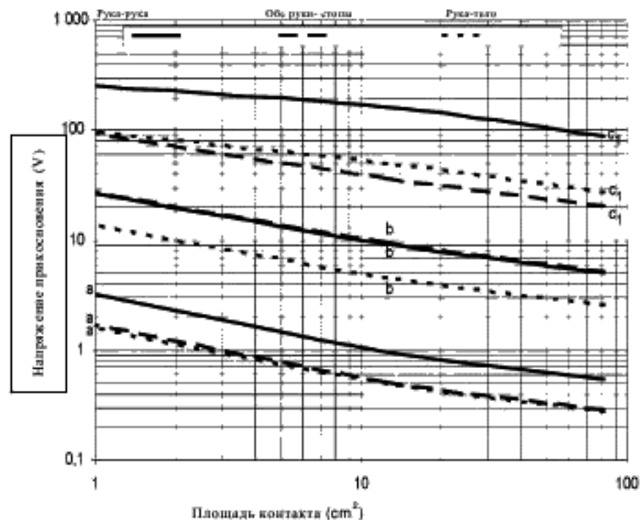
Рисунок 3 - Минимум напряжения прикосновения при переменном токе и влажных, соленых (морских) средах для тока вызывающего реакцию испуга (а), мускульную реакцию (b) и вентрикулярную фибрилляцию (c1)
