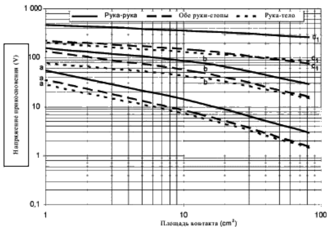
Рисунок 5 - Минимум напряжения прикосновения при постоянном токе и влажных средах для тока вызывающего реакцию испуга (а), мышечную реакцию (б) и вентрикулярную фибрилляцию (с1)
