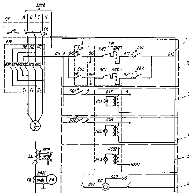
Рис. 3. Электрическая схема управления электроприводом реакторов серии РЗДПОМ: LL - дугогасящий реактор; М - электродвигатель; КМ - магнитный пускатель; QF - выключатель автоматический; RP - потенциометр; SQ - конечный выключатель; 1 - шкаф управления; 2 - местное управление; 3 - крайнее верхнее положение верхней половины стержня; 4 - крайнее нижнее положение верхней половины стержня; 5 - смещение нейтрали; 6 - датчик положения стержня
