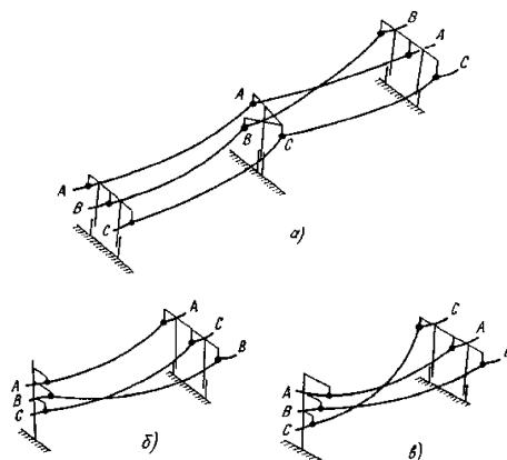
Рис. 2. Транспозиция фазных проводов на воздушных линиях
