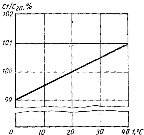
График зависимости емкости от температуры
