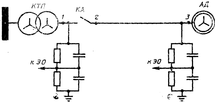
Схема коммутации низкого напряжения
