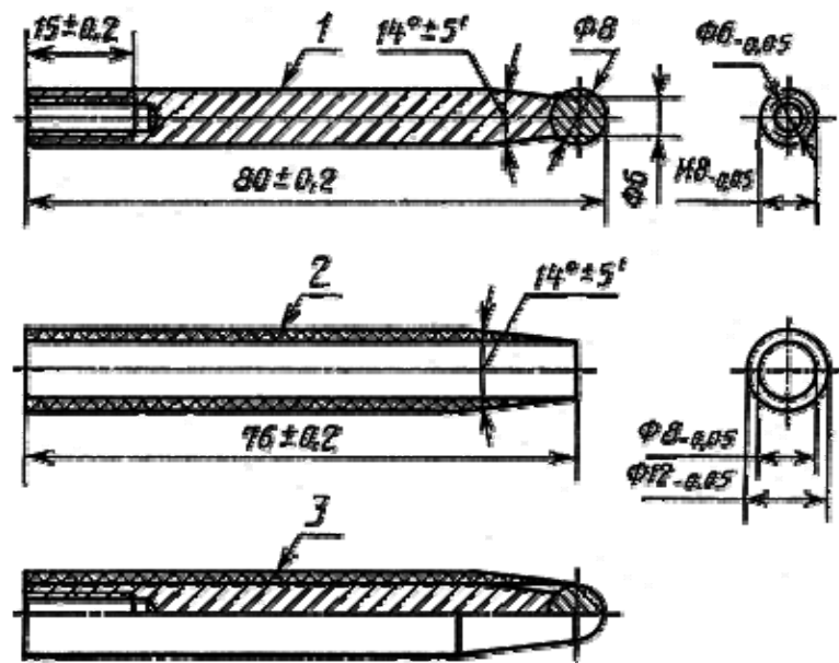
1 - латунный стержень с приваренным стальным шариком; 2 - изоляционная трубка; 3 - разрядный наконечник в сборе
