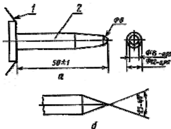
а - для воздушного разряда; б - для контактного разряда; 1 - корпус ИГ; 2 - сменный наконечник
