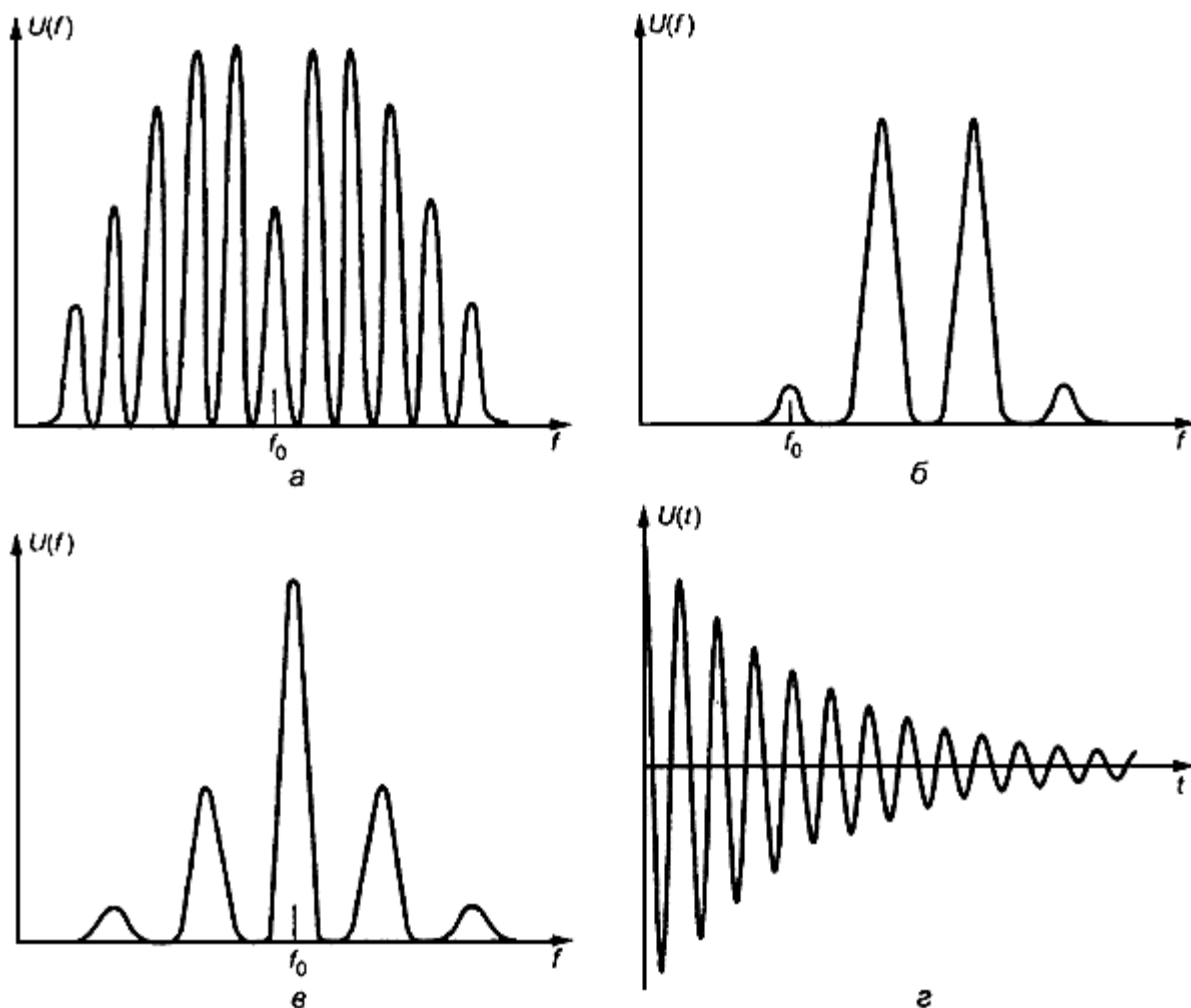
Рисунок Б.1 - Типичные характеристики излучаемых колебательных электромагнитных полей
