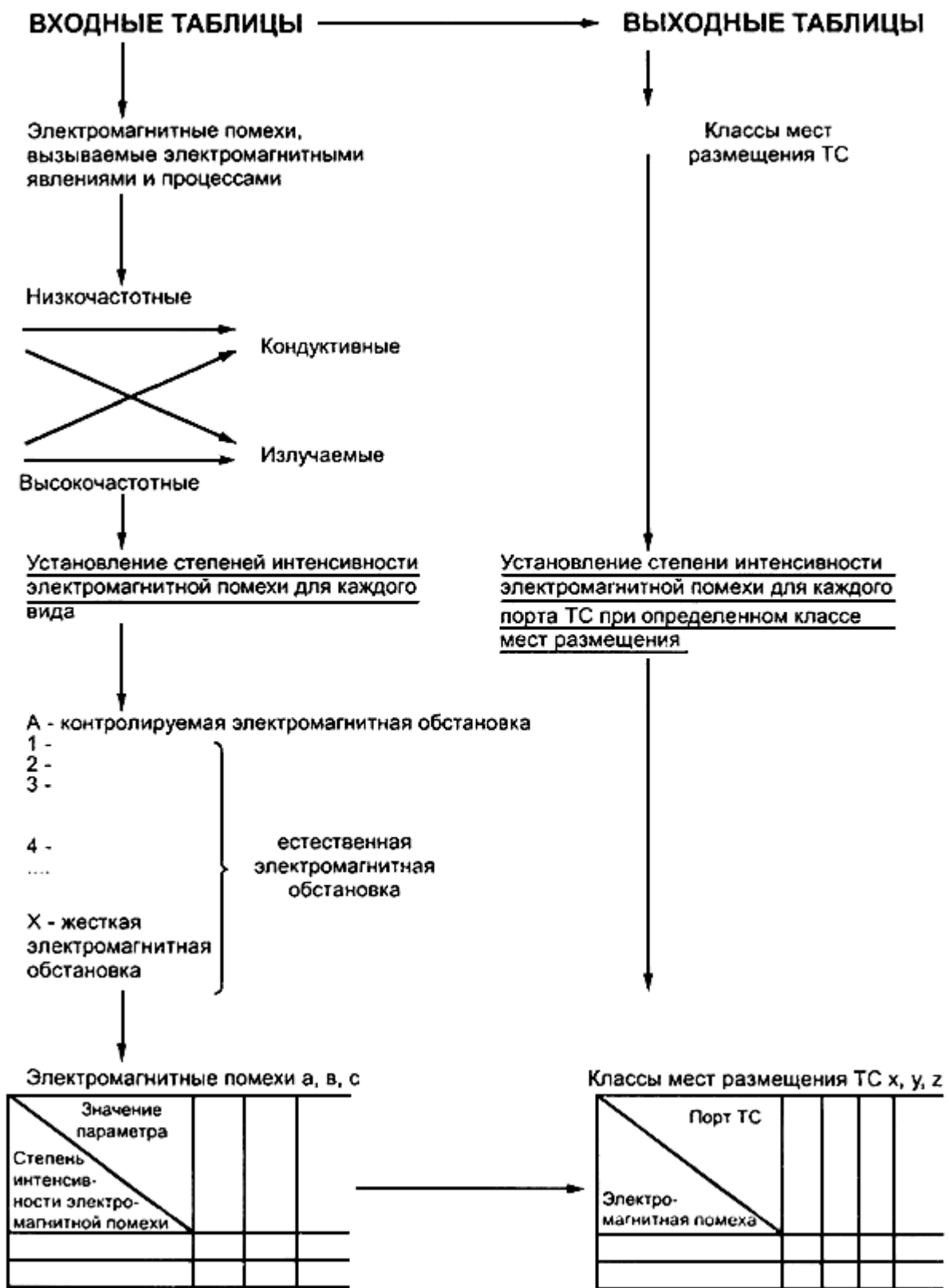
Рисунок 1 - Принцип классификации электромагнитной обстановки
