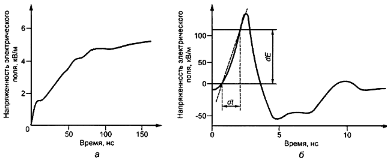
Рисунок В.1 - Типичные формы излучаемых импульсных полей
