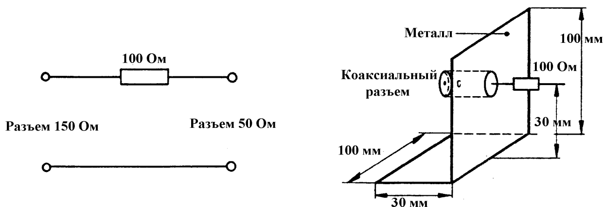
Рисунок 6 б - Схема установки для проверки полного сопротивления общего вида устройств связи / развязки
