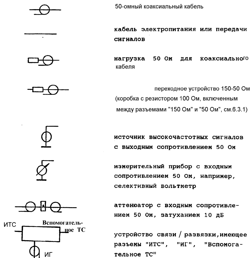
Рисунок 4а - Перечень символов, применяемых в приведенных ниже схемах рабочих мест для испытаний
