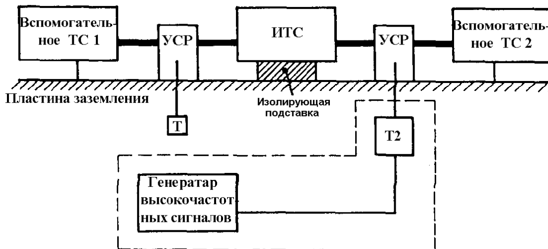
Рисунок 1а - Схема образования электромагнитных полей вблизи ИТС при протекании токов в кабелях
