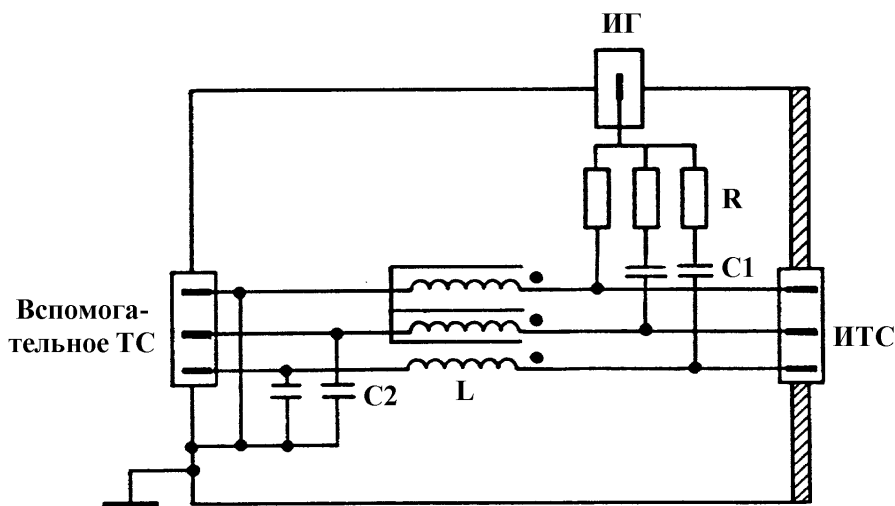
Рисунок Г.1 - Упрощенная схема устройства связи / развязки типа УСП-Н1, применяемого при вводе помехи в экранированные кабели (см. 6.2.1)
