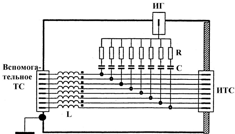
Рисунок Г.5 - Упрощенная схема устройства связи / развязки типа УСР-Т4, применяемого при вводе помехи в неэкранированные симметричные четырехпроводные линии (см. 6.2.2.2)
