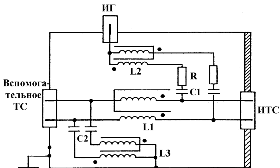
Рисунок Г.3 - Упрощенная схема устройства связи / развязки типа УСП-НС2, применяемого при вводе помехи в неэкранированные несимметричные линии (см. 6.2.2.3)
