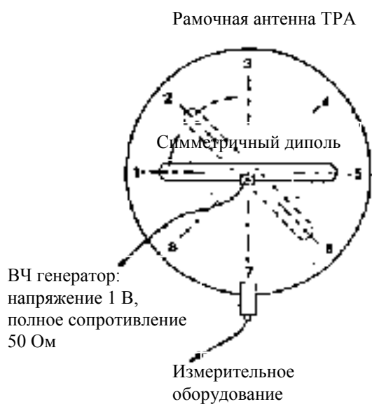
Рисунок Б.4 – Испытательная установка для оценки ТРА
