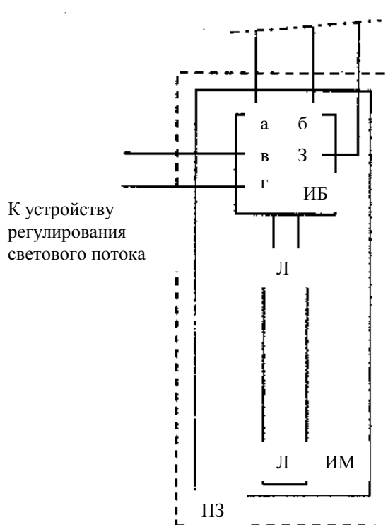
Рисунок 6б – Отдельные балласты для люминесцентных и других разрядных ламп
