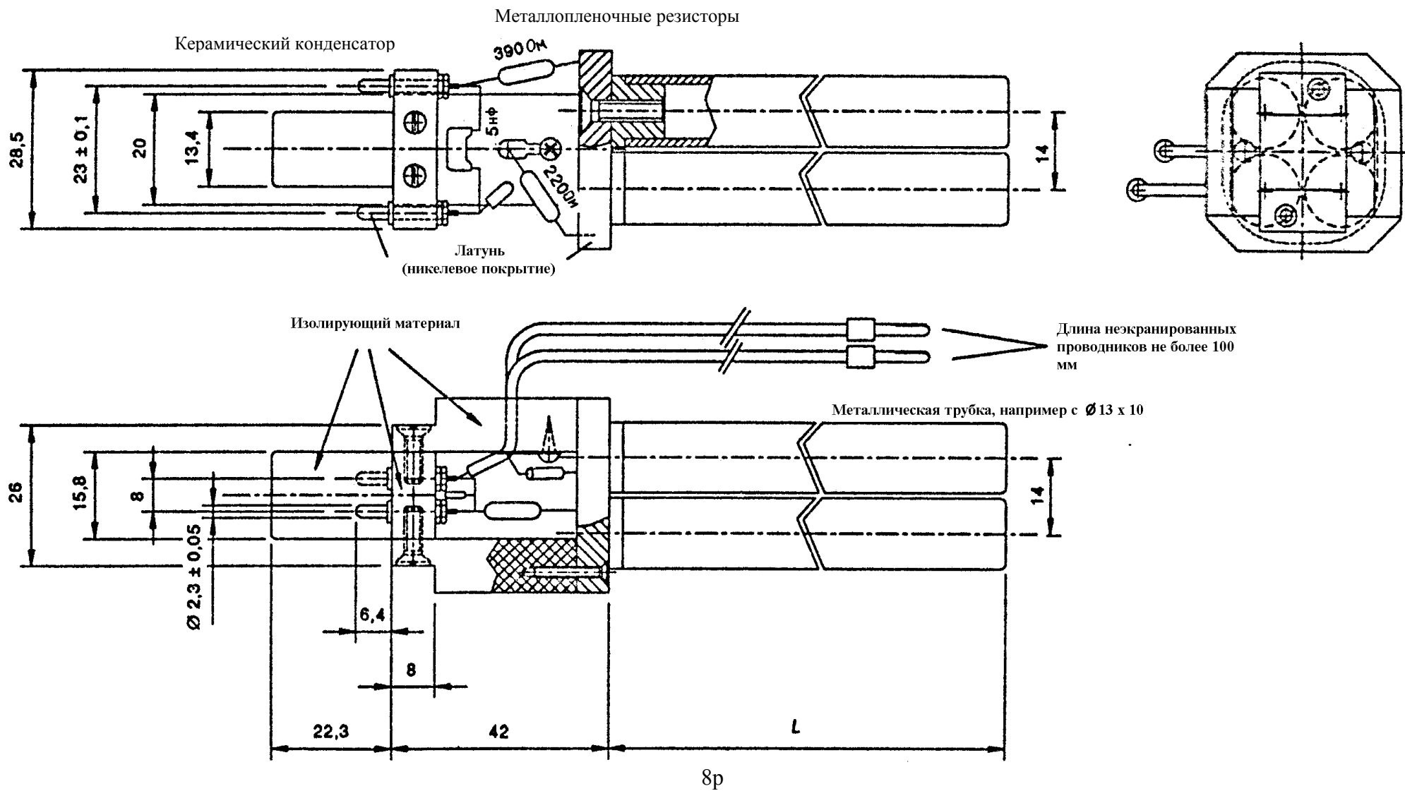
Рисунок 4е – Эквивалент одноцокольной четырехтрубчатой линейной люминесцентной лампы с диаметром трубок 12 мм
