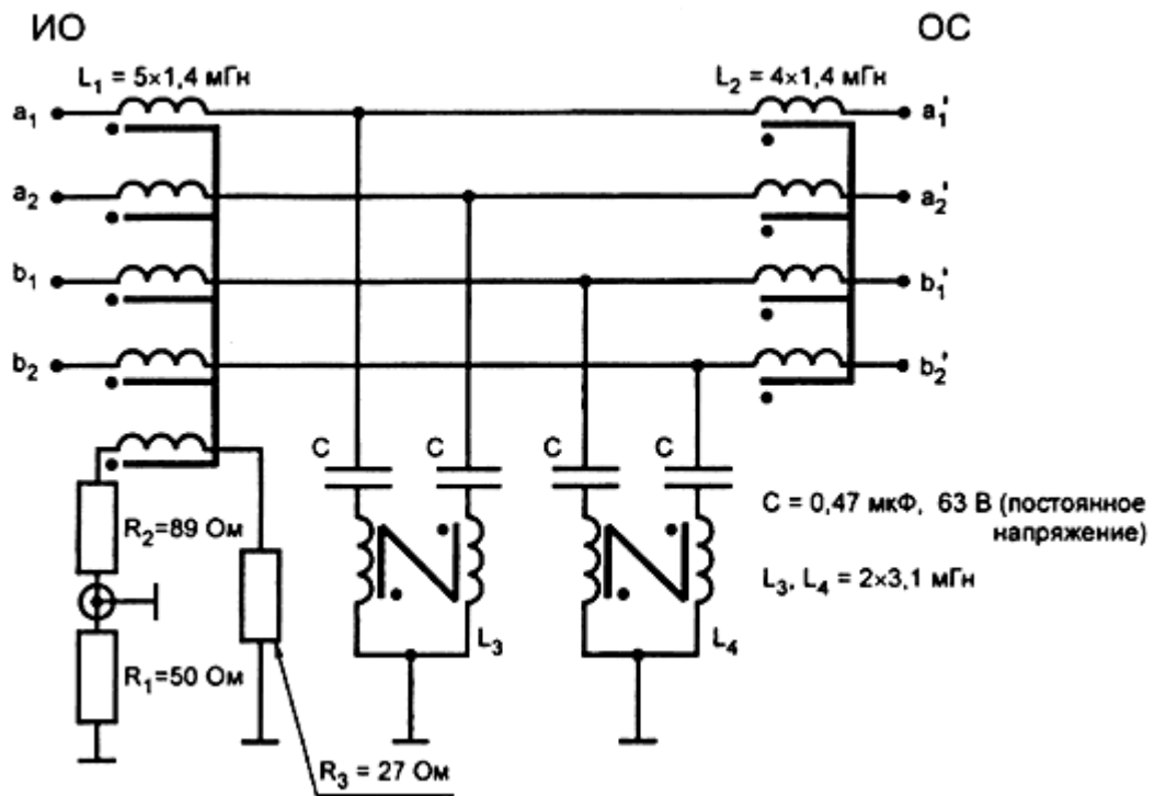
Рисунок В.2 - Эквивалент полного сопротивления сети с большим затуханием продольного перехода для применения с двумя незранированными симметричными парами
