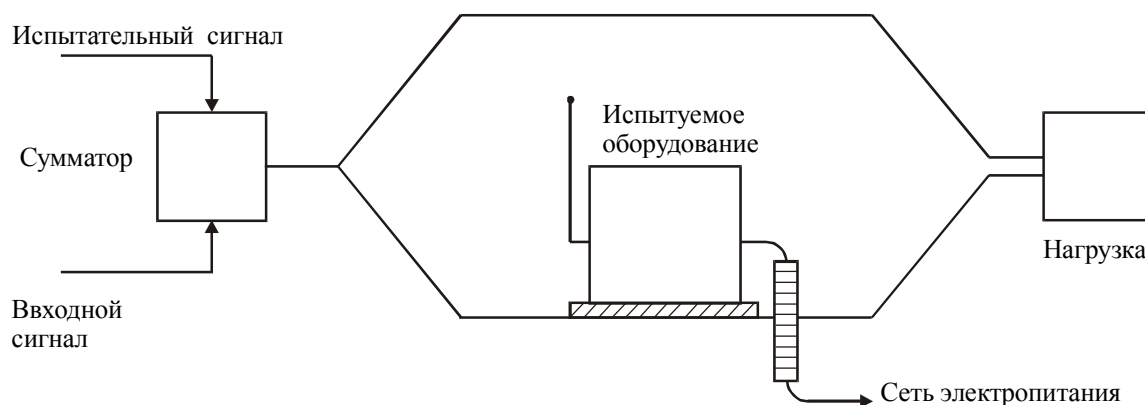
Рисунок 2 – Схема расположения оборудования со встроенной антенной, не имеющего входных антенных зажимов, при воздействии электромагнитного поля в полосе частот от 0,15 до 150 МГц
