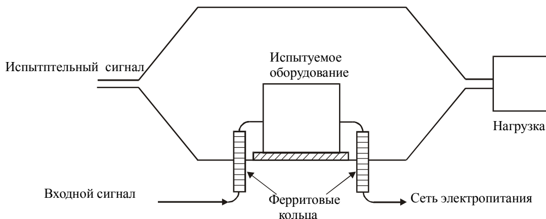
Рисунок 1 – Схема расположения оборудования при воздействии электромагнитного поля в полосе частот от 0,15 до 150 МГц
