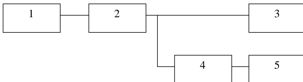
1 – генератор сигналов звуковой частоты; 2 - испытуемый усилитель звуковой частоты; 3 – громкоговоритель или эквивалент нагрузки; 4 - полосовой фильтр ; 5 – вольтметр переменного тока
