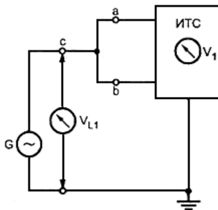
Рисунок 6 - Измерение степени подавления общего несимметричного напряжения
