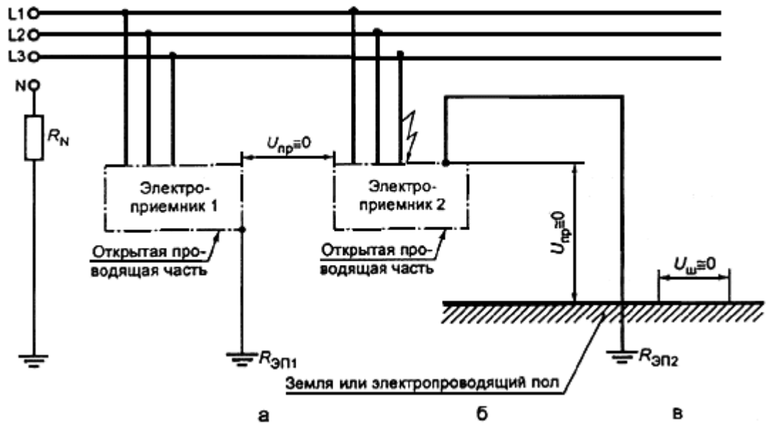
Рисунок В.12 - Сеть IT с заземлением нейтрали источника питания через сопротивление с однофазным замыканием на корпус
