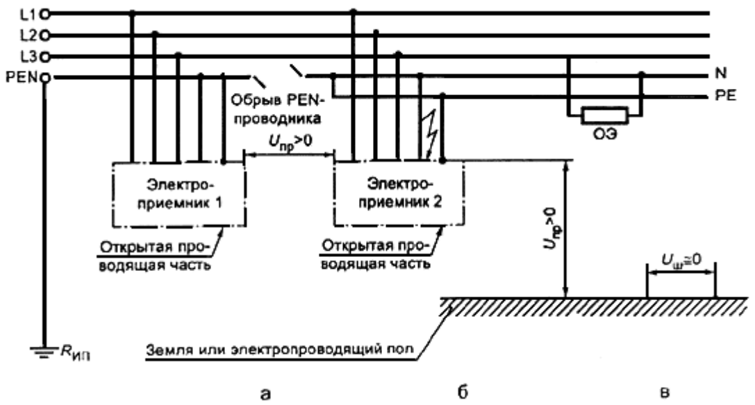
Рисунок В.7 - Сеть TN-C-S с обрывом PEN-проводника
