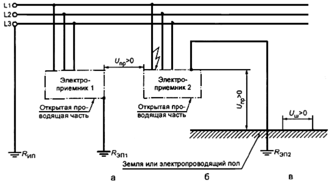
Рисунок В.11 - Сеть ТТ без нулевого рабочего проводника с однофазным замыканием на корпус
