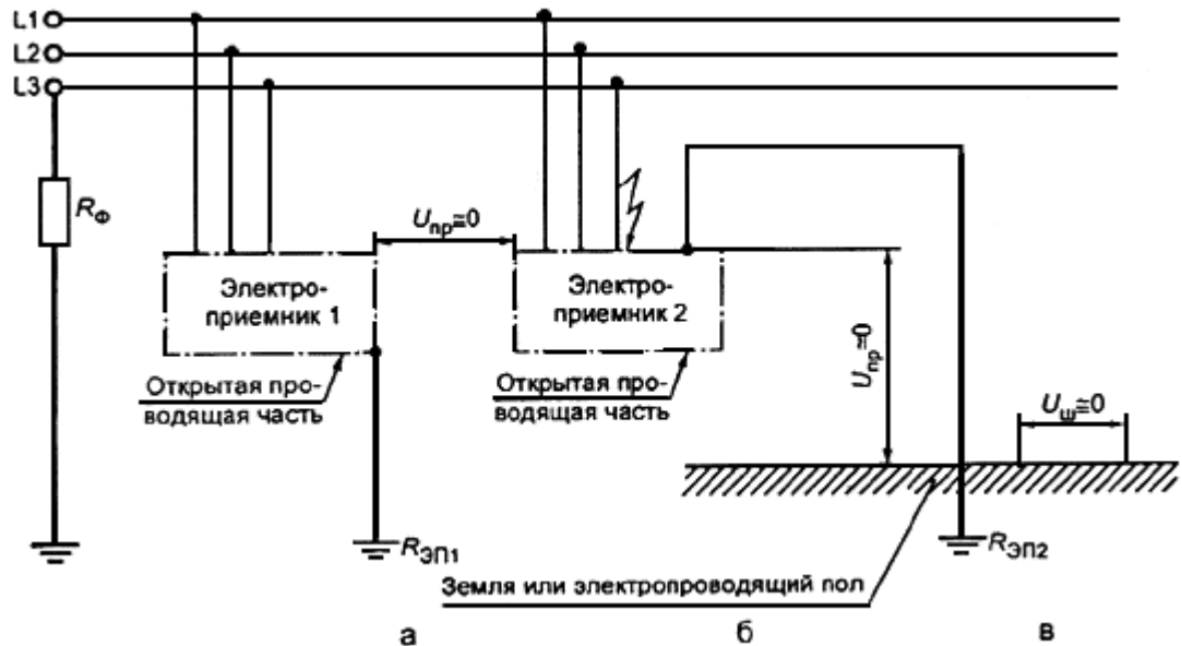
Рисунок В.13 - Сеть IT с заземлением фазы источника питания через сопротивление с однофазным замыканием на корпус
