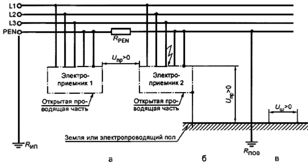
Рисунок В.3 - Сеть TN-C с однофазным замыканием на корпус
