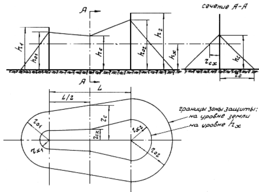
Рис. 3.3. Зона защиты двух стержневых молниеотводов разной высоты.
