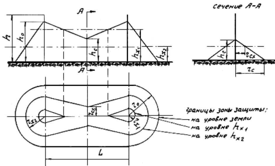
Рис. 3.2. Зона защиты двойного стержневого молниеотвода
