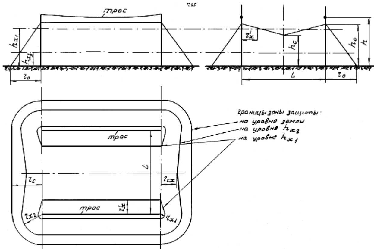
Рис. 3.6. Зона защиты двойного тросового молниеотвода
