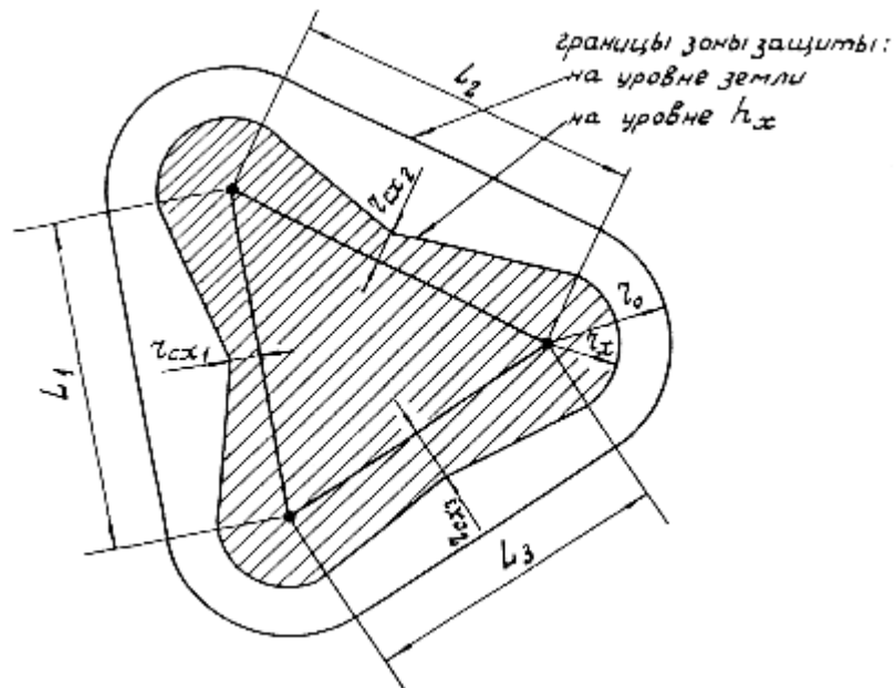
Рис. 3.4. Зона защиты (в плане) многократного стержневого молниеотвода
