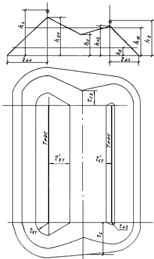
Рис. 3.7. Зона защиты двух тросовых молниеотводов разной высоты
