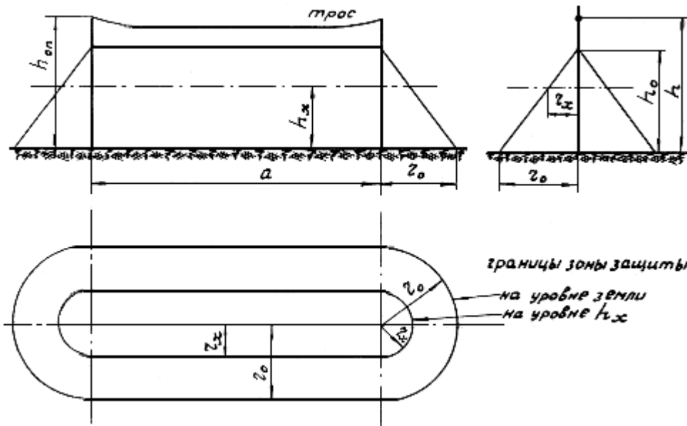
Рис. 3.5. Зона защиты одиночного тросового молниеотвода
