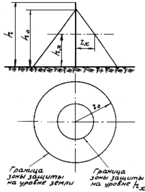
Рис. 3.1. Зона защиты одиночного стержневого молниеотвода
