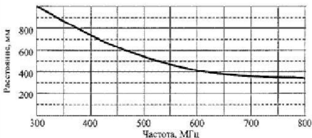
Рисунок П 2.1. Расстояния, на которых следует проводить измерения ППЭ ЭМП от подвижных станций, работающих в диапазоне частот \geq 300 —800 МГц. При этом контролируемый уровень ППЭ ЭМП в диапазоне частот \geq 300 —2400 МГц не должен превышать 3 мкВт/см 2 , что обеспечивает соблюдение требований п. 4.1 настоящих Санитарных правил.
