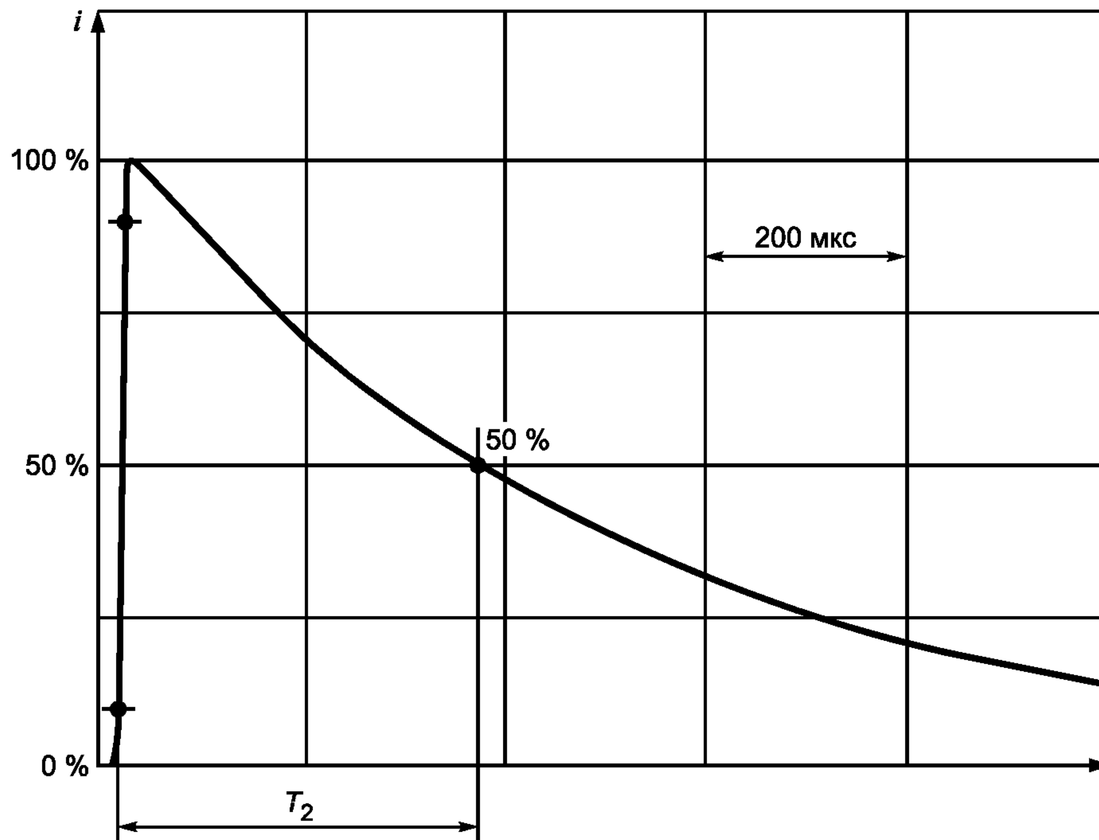
Рисунок В.2 — Кривая хвоста тока положительного импульса
