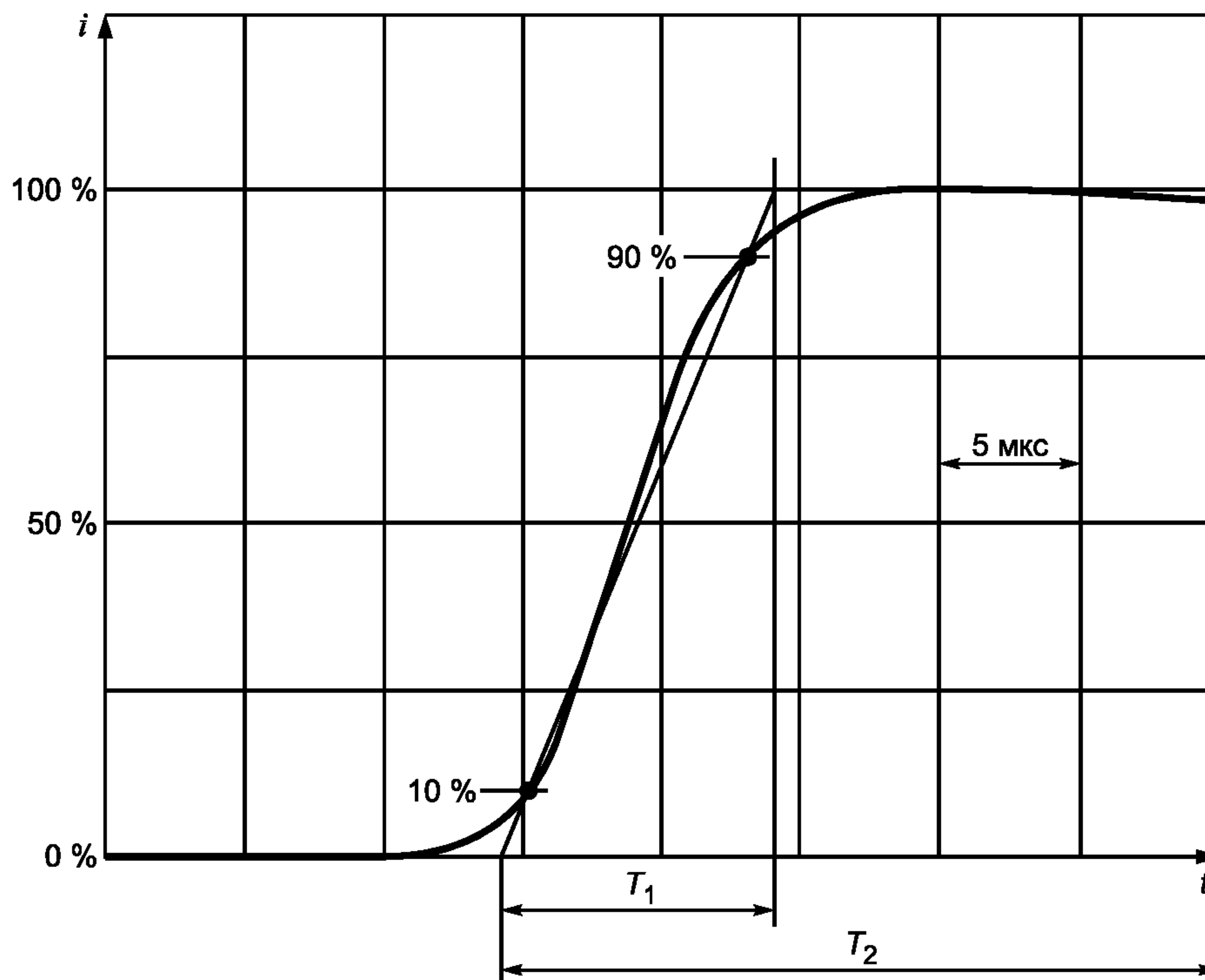
Рисунок В.1 — Кривая нарастания тока положительного импульса
