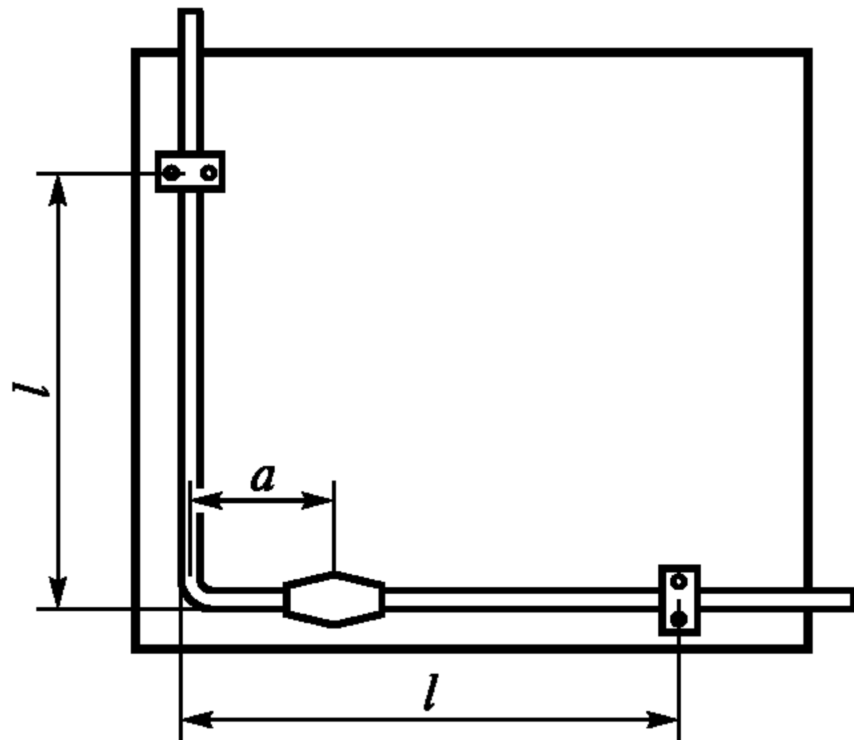
Рисунок D.2 — Конфигурация проводников в LPS
