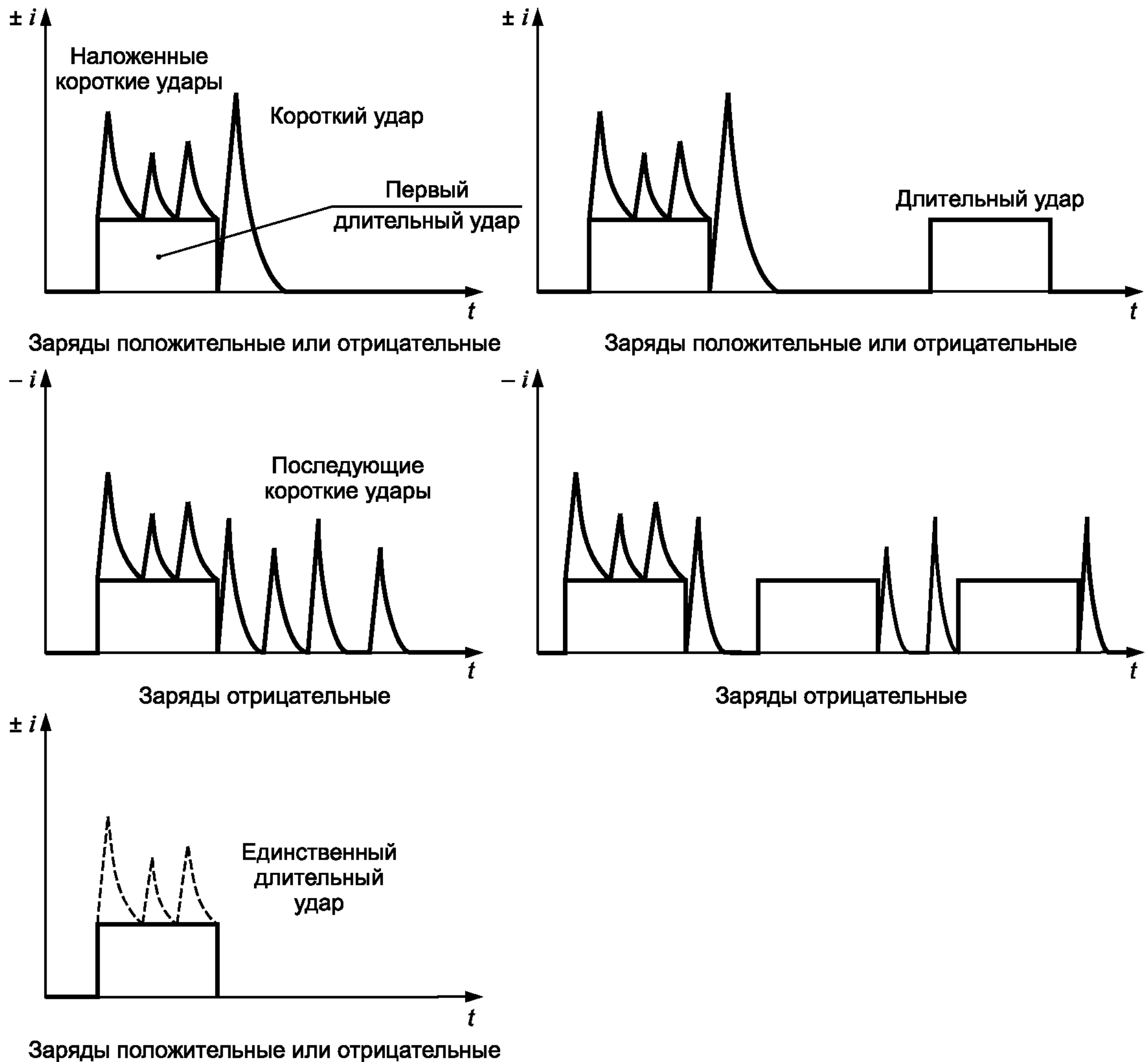
Рисунок А.4 — Типичные компоненты восходящих разрядов молнии для зданий средней высоты и/или высотных зданий (сооружений)
